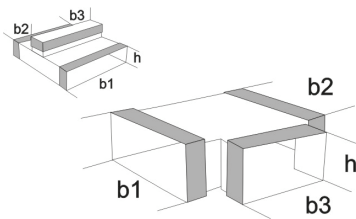
Zwischenstück/Endstück
