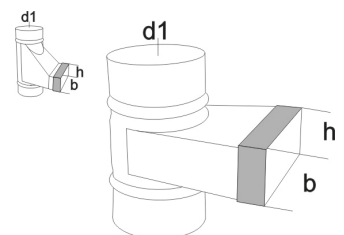
Abzweig
