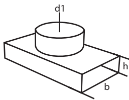
Kanalschalldämpfer
